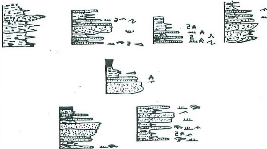
Fig. - 1 Facies y Asociaciones de facies en las Formaciones del Precámbrico
